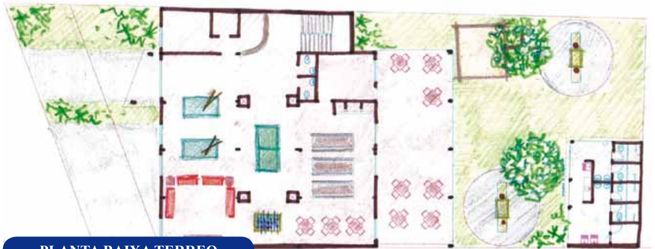
PLANTA BAIXA TERREO
